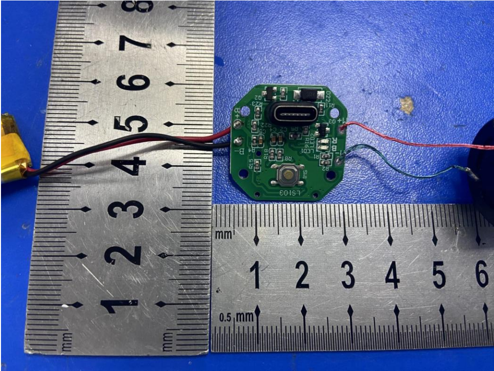
图片.7. PCB 视图-RP-MA09 C
