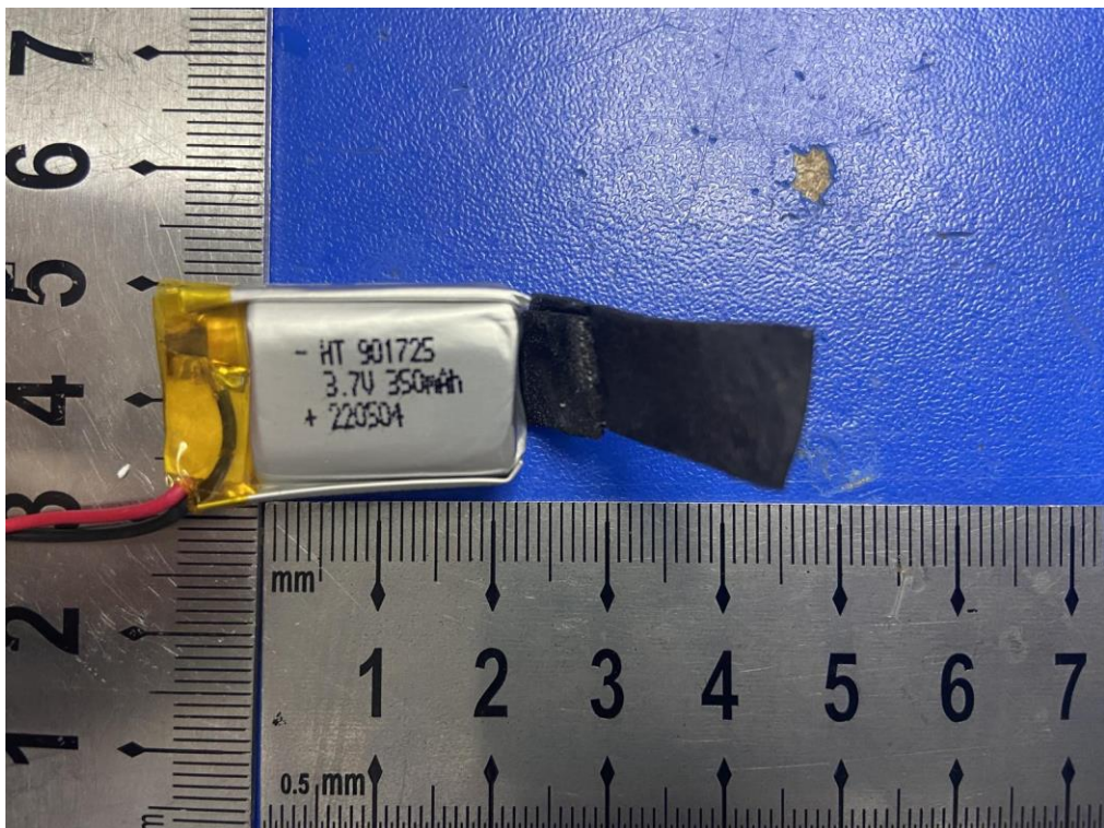
图片.6. 电池视图-RP-MA09 C
