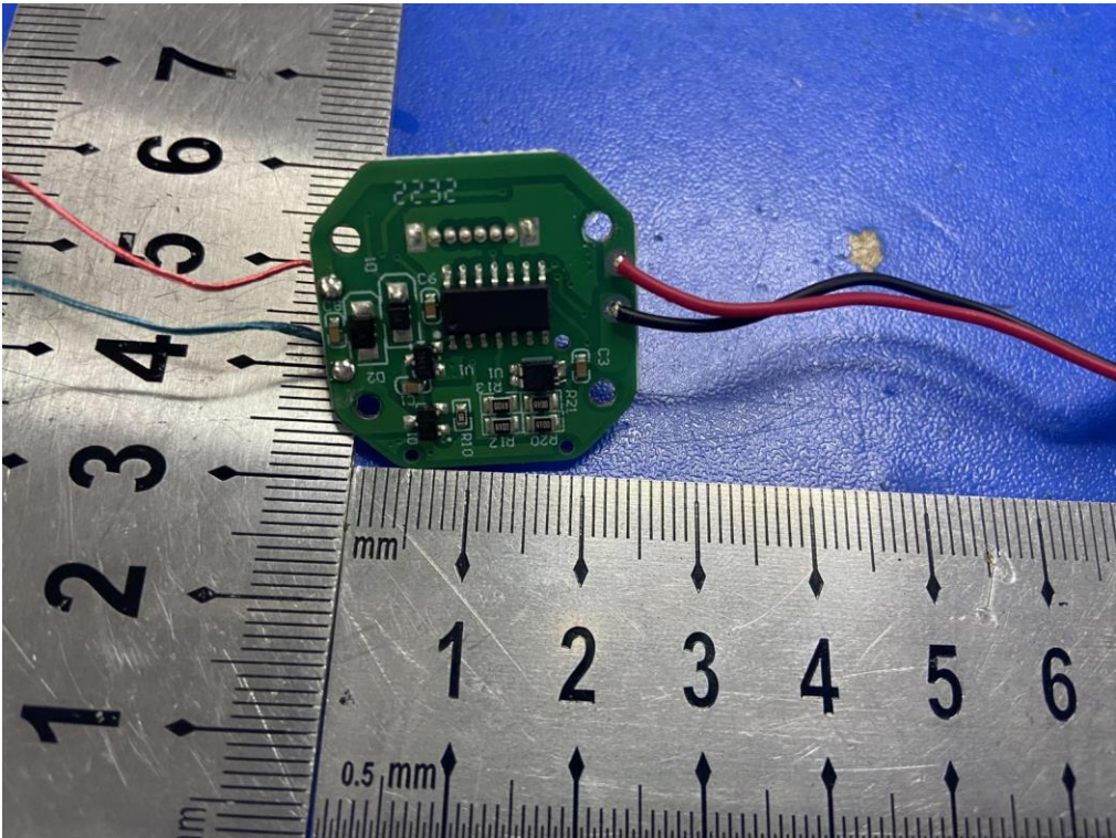
图片.8. PCB 视图-RP-MA09 C
