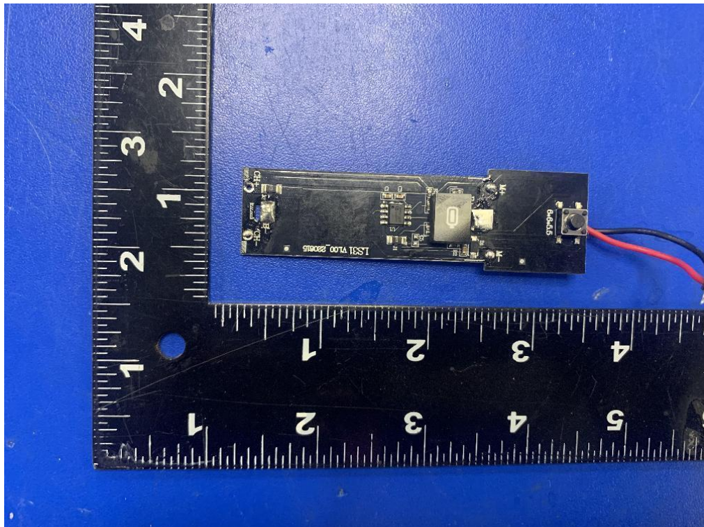
图片.12. PCB 正面视图
