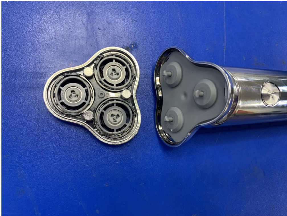
图片.7. 刀头拆分视图 (RS366)
