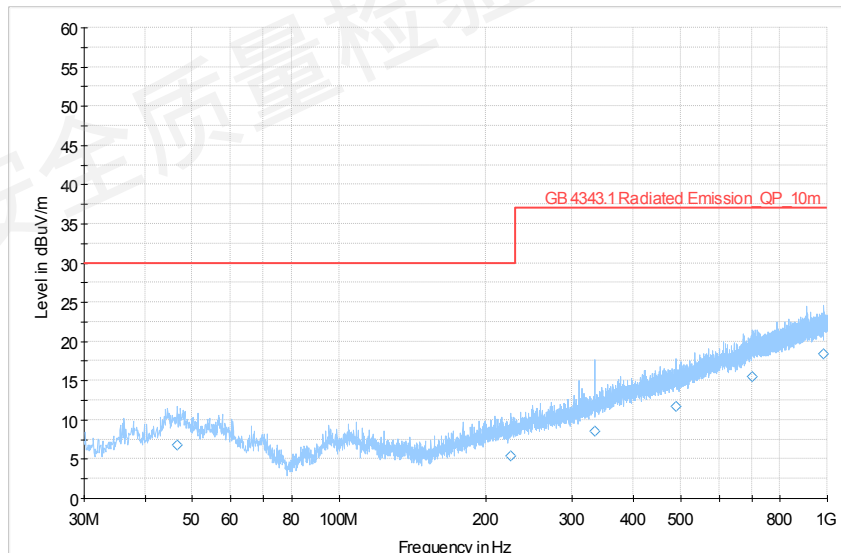
辐射骚扰 (30MHz~1GHz) 检验数据-水平极化
