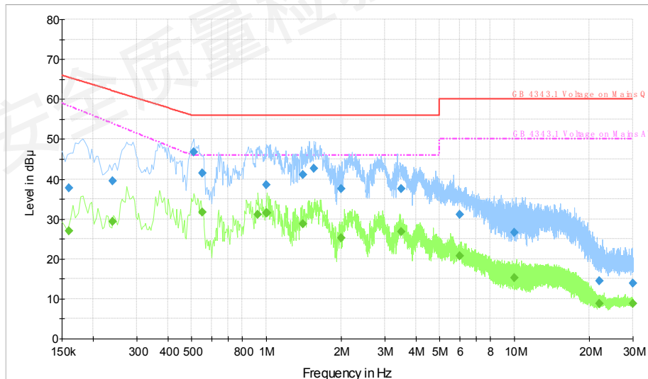
骚扰电压检验数据
