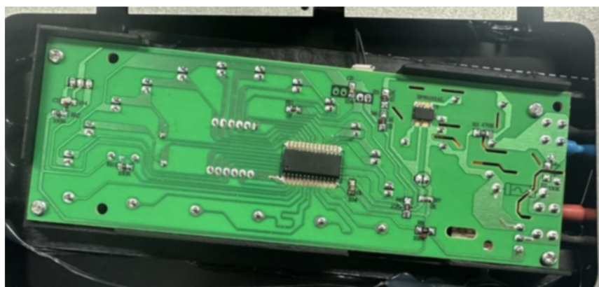
PCB 板背面
