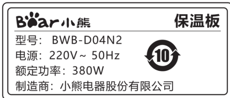
铭牌
