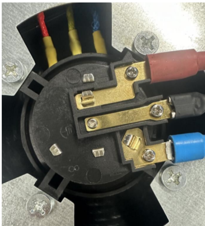
内部连接
