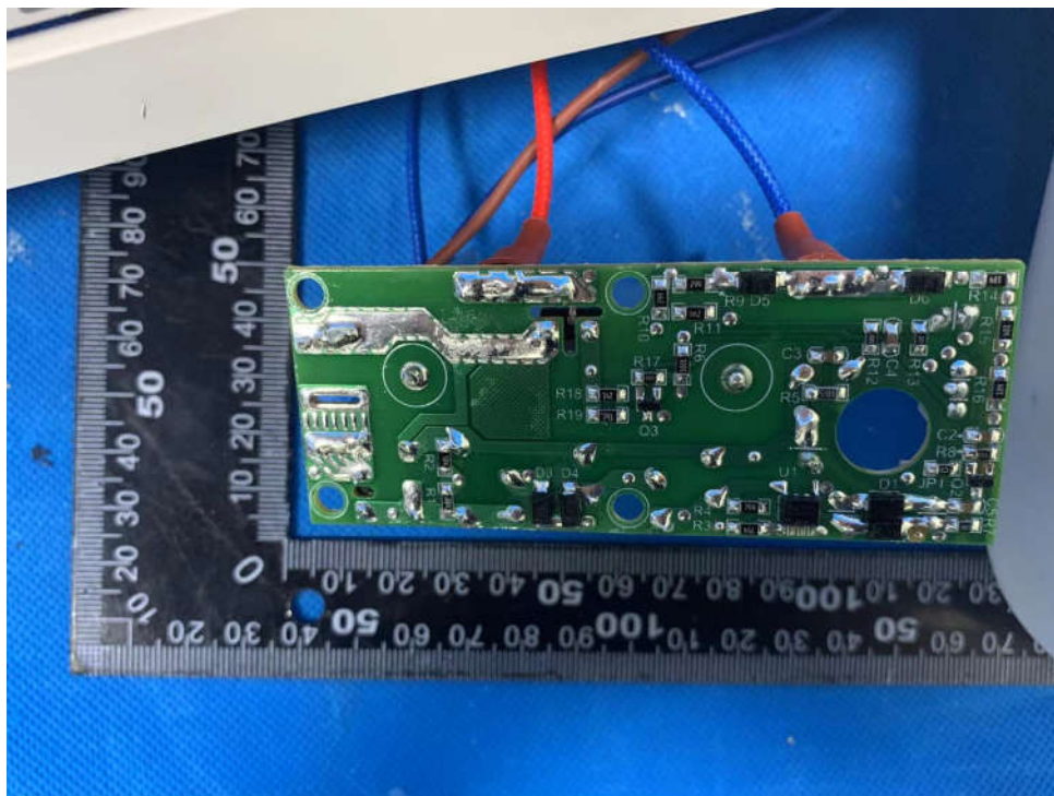
主检型号 DZ01 电源 PCB(反面)
