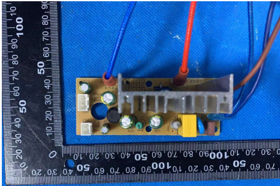
主检型号 DZ01 电源 PCB(正面)
