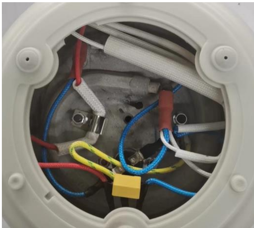
变更前 (热熔断体固定使用金属片压紧)
