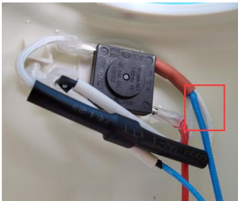
变更后 (氙灯线的一端接到档位开关)
