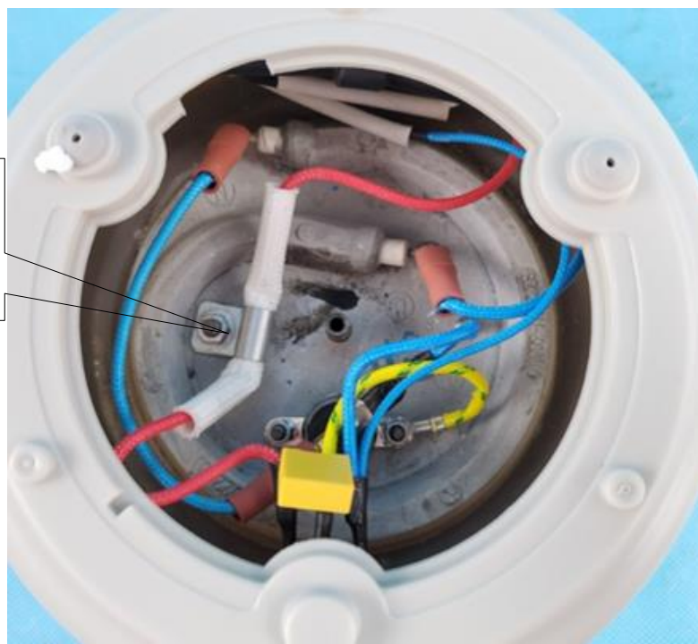
变更后 (热熔断体固定使用金属片包围后双压紧)
