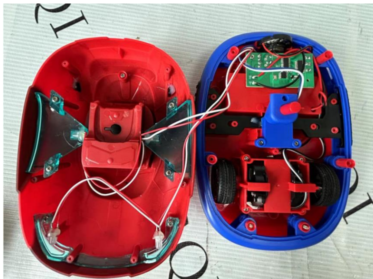
差异：757-B067 的内部结构图（车内部结构一致）
